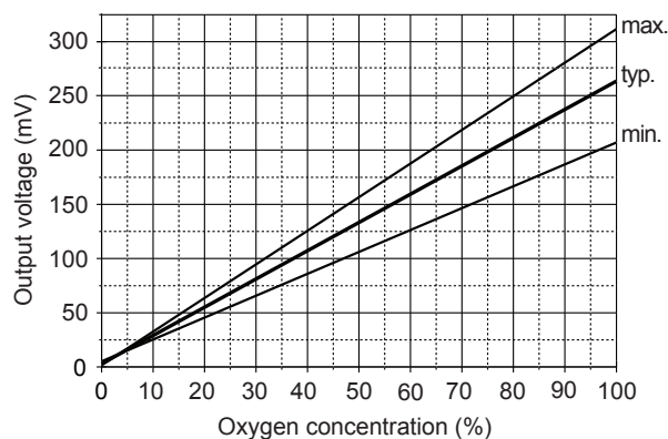
Fig. 3b - KE-50 sensitivity characteristics
